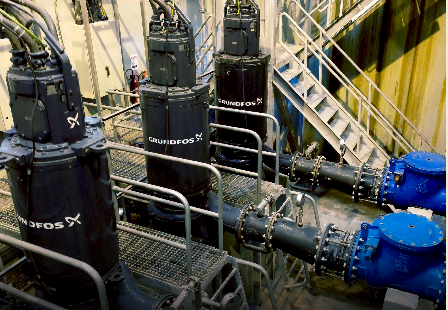
S-Pumpen von Grundfos bei einer der Pumpstationen der RAKWA in Ras Al Khaimah, VAE.
